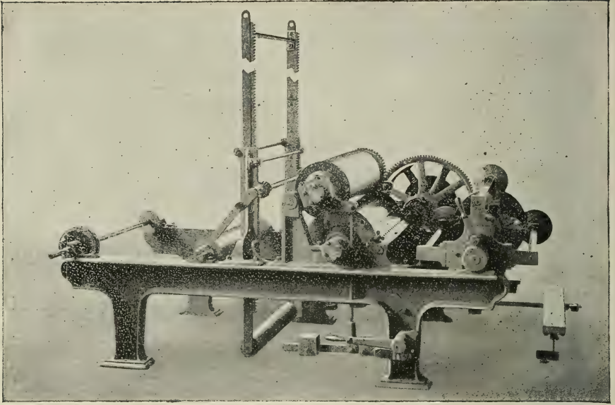
FIG. 120.—Tar Saturator.
